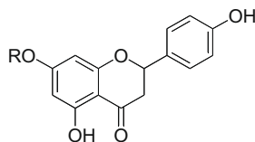
R = neohesperidosyl 5
